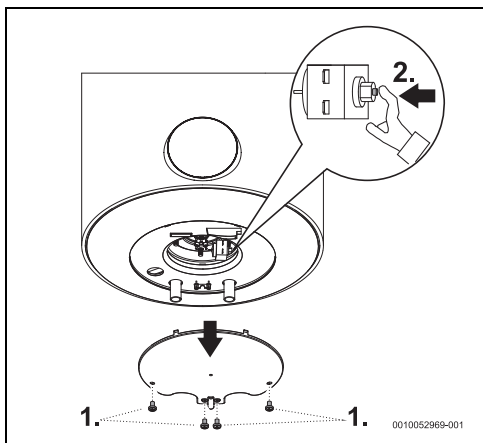
Fig. 11 Termostato de seguridad
