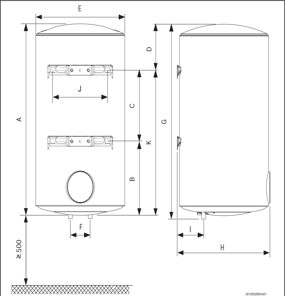
Fig. 2 Mediciones en mm (montaje en pared, instalación vertical)
